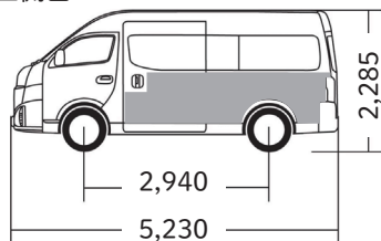
左側面
