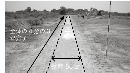
連続地中壁工実施状況
