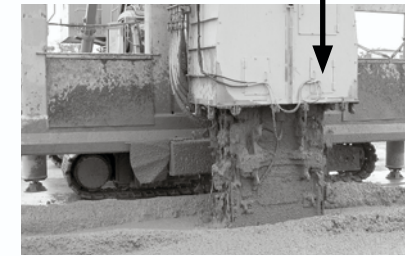
TRD 工法実施状況
