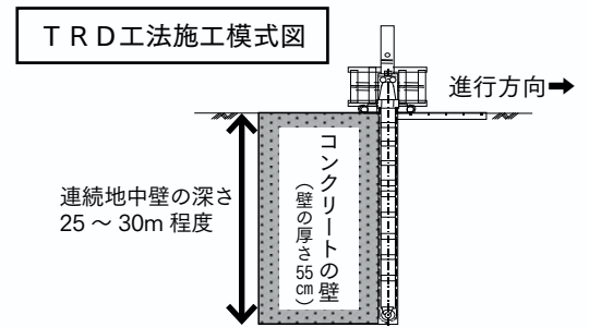
連続地中壁工実施状況
