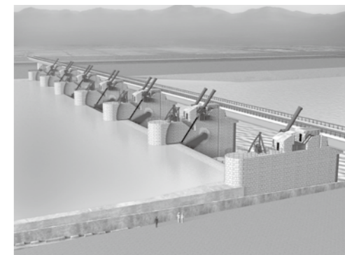
大河津可動堰完成イメージパース (右岸高水敷上空より)
