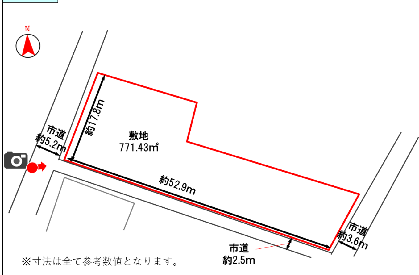
配置図
